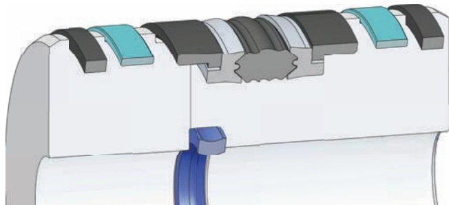
A403 Kapak Keçesi
