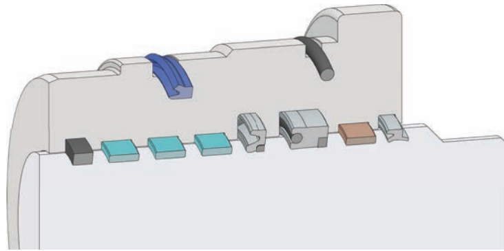
A405 Statik Sızdırmazlık Keçesi
