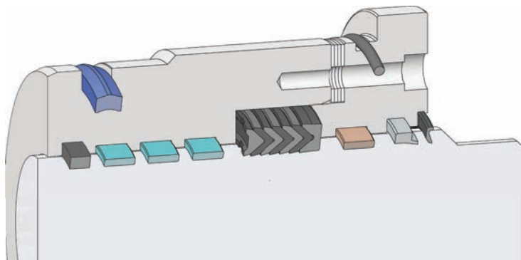
A404 Kapak Keçesi
