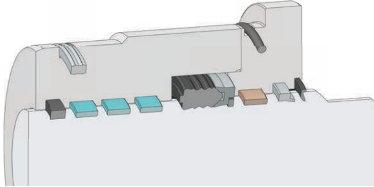
A406 Statik Sızdırmazlık Keçesi
